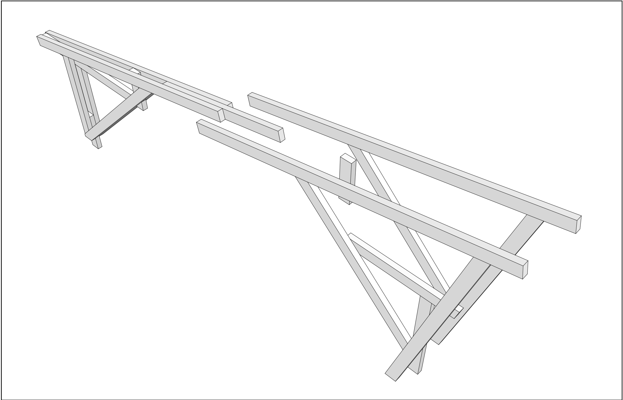
[6] Detalhe - TESOURA (EXPLODIDA)
